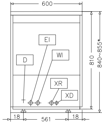
前视图 FRONT-VIEW
